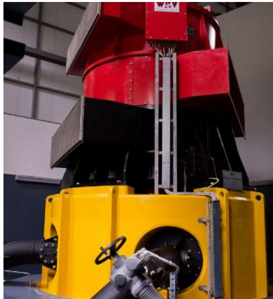
Turbina Pelton de eje vertical con 5 inyectores
